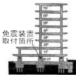
中間階免震工法(地下1階柱頭)
